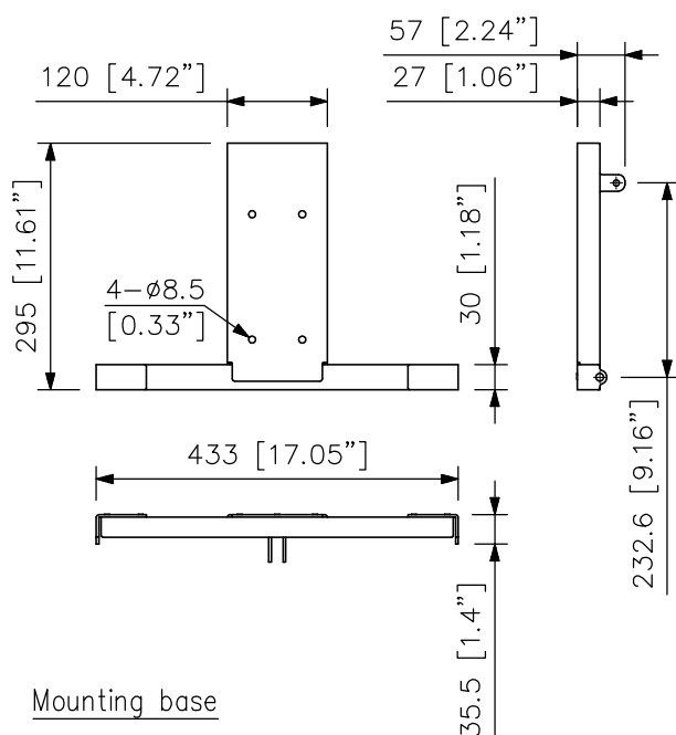
T-bracket (scale: 1/10)
